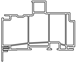
1/2" FLUSH FIN
